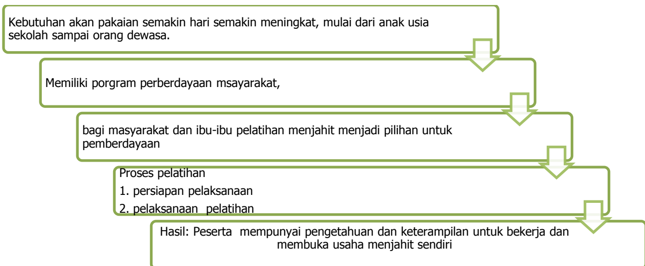
Gambar 1. Kerangka Pikir
